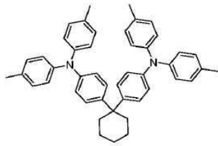
TAPC
