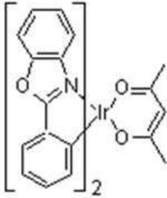
bo 2 Ir(acac) (525nm)
