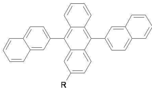
DNA/MADN/TBADN
