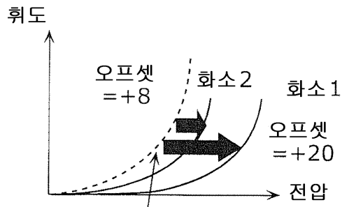
대표 전류-전압 특성
