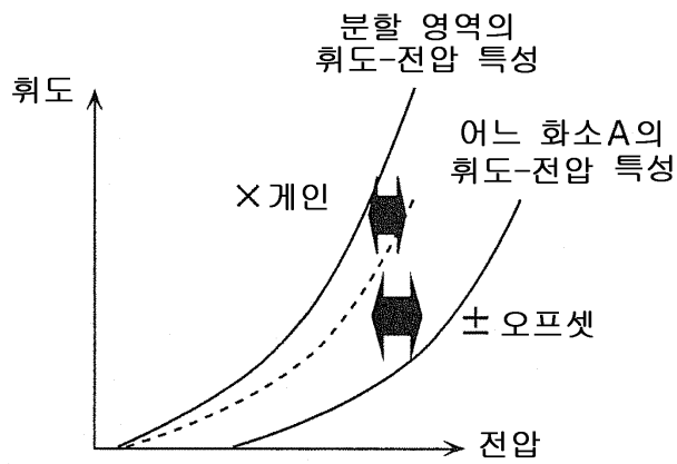
전압 계인과 오프셋을 구하는 경우
