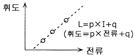
(b) 분할 영역마다의 EL의 전류-휘도 특성
