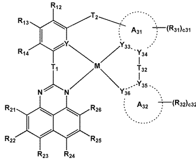
<화학식 1c>
