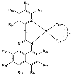
<화학식 1c>
