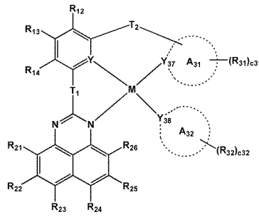
<화학식 1d>
