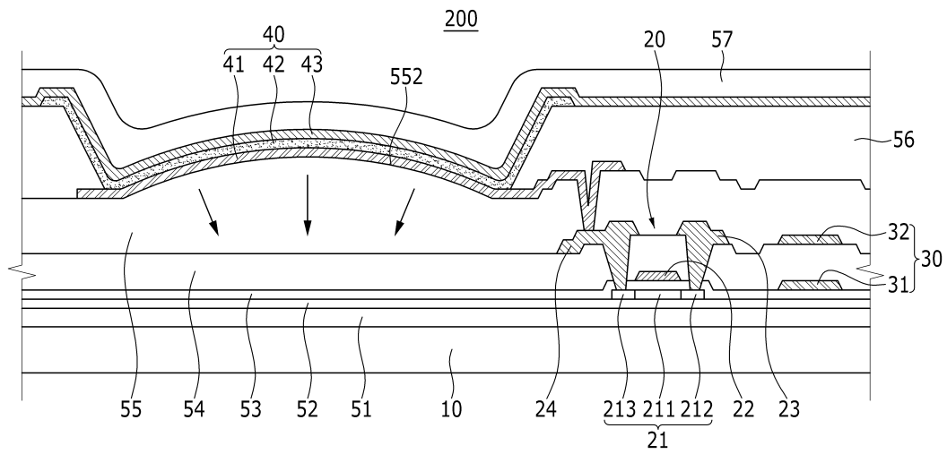
도면4
