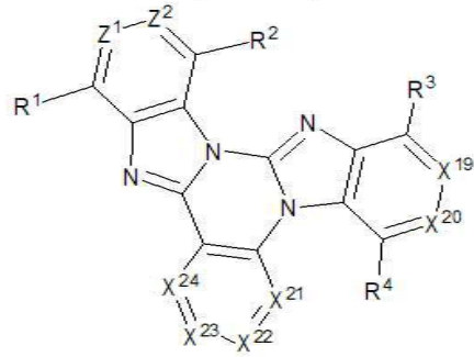
[구조식 5]
