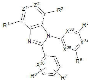
[구조식 9]
