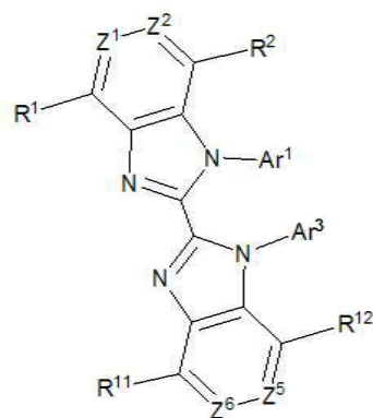
[구조식 9]
