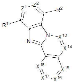
[구조식 6]
