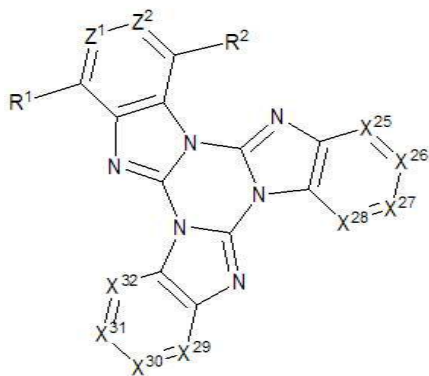
[구조식 8]
