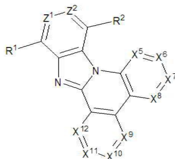
[구조식 3]
