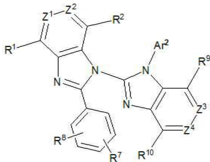
[구조식 8]
