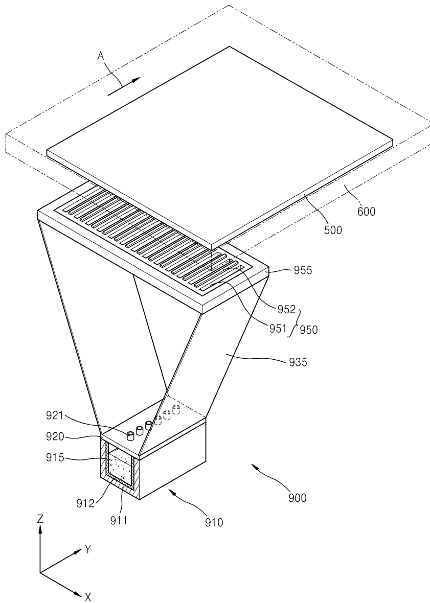
도면12
