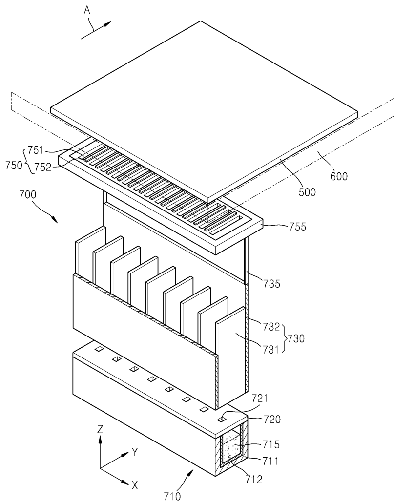
도면8
