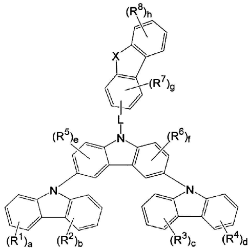
[화학식 1-1]
