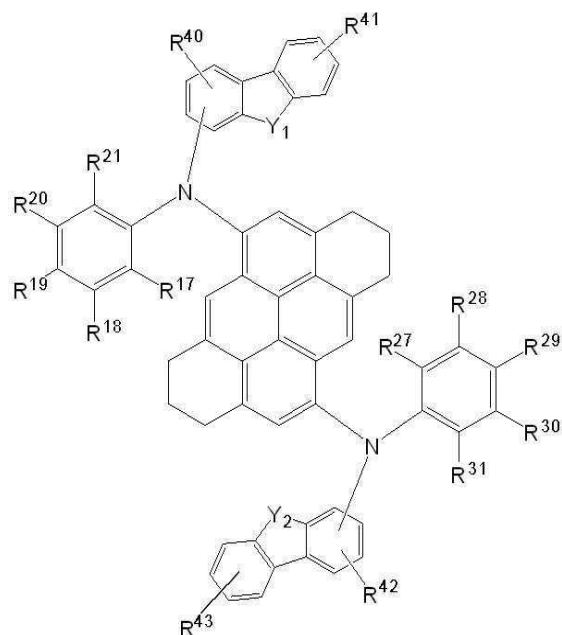
[구조식 4]
