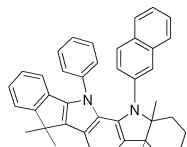
[화학식 44]
