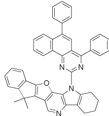
[화학식 27]
