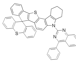
[화학식 65]
