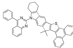
[화학식 59]
