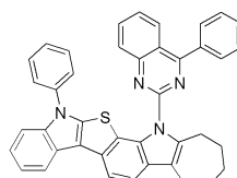
[화학식 77]
