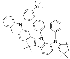
[화학식 56]
