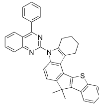
[화학식 71]
