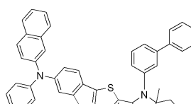
[화학식 46]
