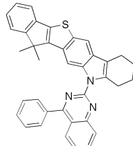
[화학식 64]
