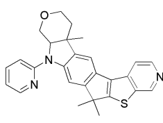
[화학식 79]
