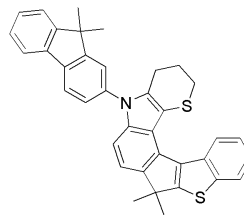
[화학식 80]
