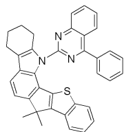
[화학식 66]
