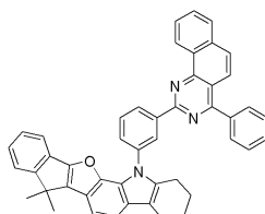
[화학식 33]
