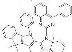
[화학식 44]
