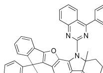
[화학식 45]
