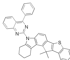
[화학식 68]
