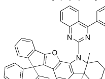
[화학식 45]
