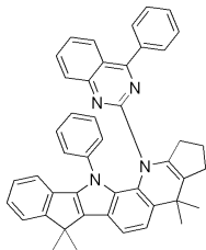
[화학식 75]
