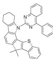
[화학식 66]
