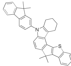
[화학식 74]
