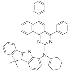
[화학식 28]
