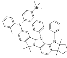
[화학식 55]
