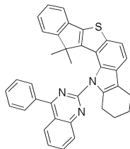
[화학식 63]
