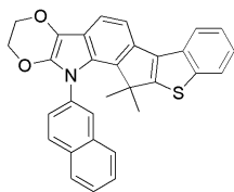
[화학식 78]
