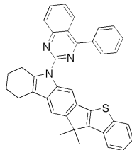
[화학식 67]
