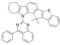
[화학식 69]
