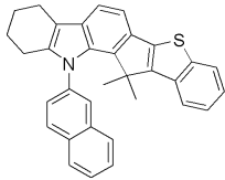
[화학식 72]
