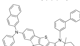
[화학식 46]
