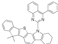
[화학식 9]
