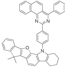
[화학식 30]
