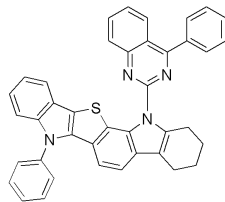
[화학식 13]
