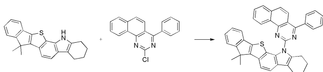
[화합물 25]
