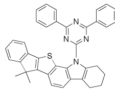
[화학식 4]
