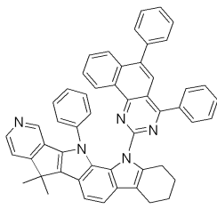
[화학식 26]
