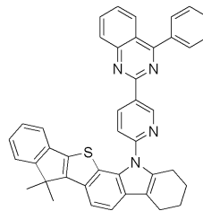
[화학식 37]
