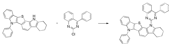
[화합물 13]
