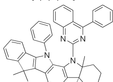
[화학식 44]
