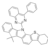
[화학식 39]
