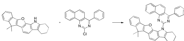
[화합물 24]
