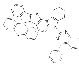
[화학식 65]
