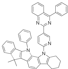
[화학식 35]
