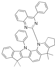
[화학식 75]
