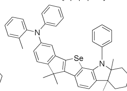
[화학식 53]
