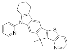
[화학식 73]
