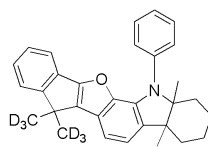
[화학식 52]
