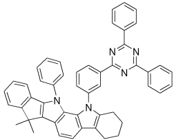
[화학식 8]
