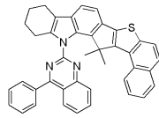
[화학식 58]
