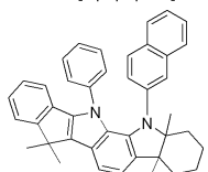
[화학식 44]
