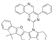
[화학식 42]
