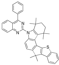
[화학식 60]
