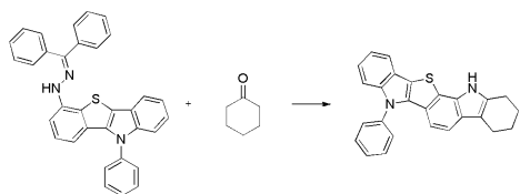
[중간체 2-f]
