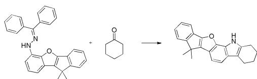
[중간체 3-h]
