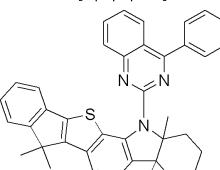
[화학식 46]
