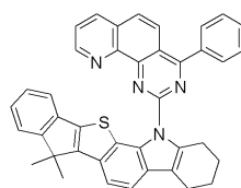
[화학식 40]
