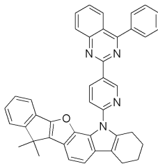
[화학식 36]
