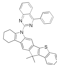
[화학식 67]
