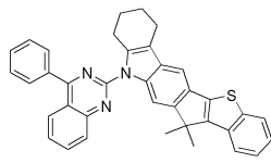
[화학식 70]
