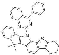
[화학식 39]
