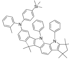
[화학식 56]
