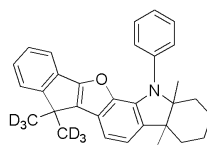
[화학식 52]
