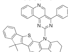
[화학식 43]
