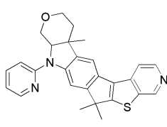
[화학식 79]
