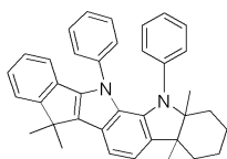
[화학식 51]
