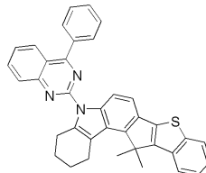
[화학식 68]
