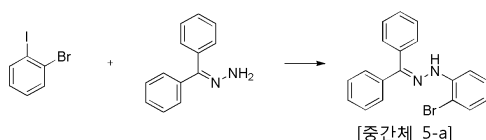
[중간체 5-a]
