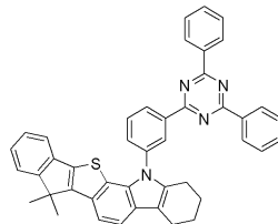
[화학식 10]
