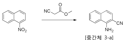
[중간체 3-a]
