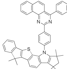
[화학식 31]
