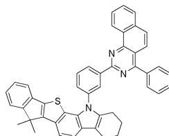
[화학식 34]
