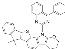
[화학식 76]
