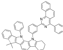
[화학식 32]
