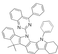
[화학식 38]
