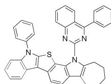
[화학식 77]
