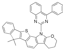
[화학식 76]
