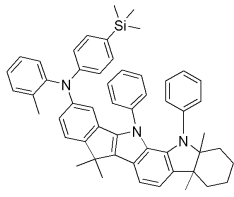
[화학식 54]
