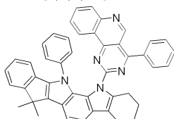
[화학식 41]
