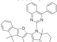
[화학식 45]
