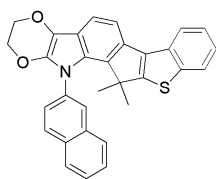
[화학식 78]
