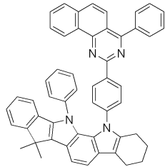
[화학식 29]
