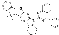
[화학식 61]
