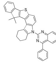
[화학식 62]
