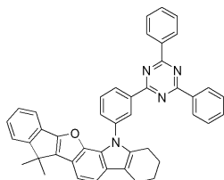
[화학식 9]
