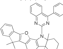
[화학식 45]
