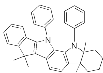
[화학식 51]
