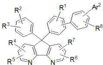
[구조식 2]
