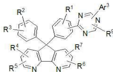
[구조식 3]
