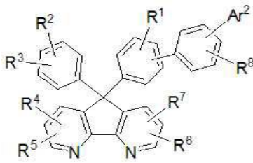
[구조식 4]
