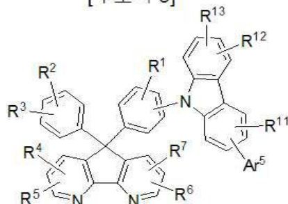
[구조식 5]
