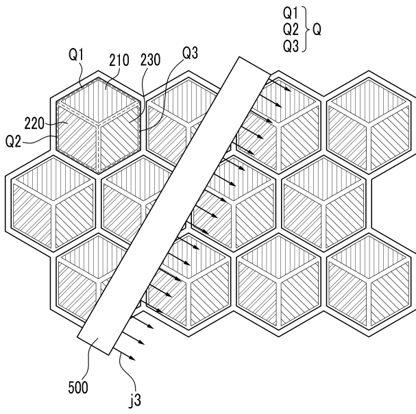
도면17
