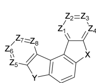
[화학식 5]
