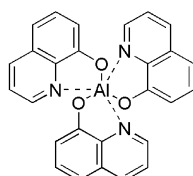
Alq
