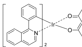
(piq) 2 Ir(acac)
