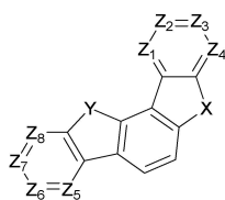
[화학식 4]
