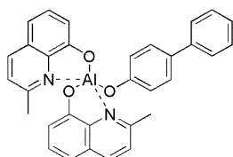
BALq
