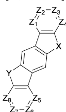
[화학식 4]
