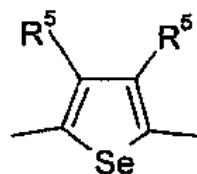
셀레노펜-2,5-디일,
