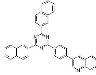
[화학식 14]
