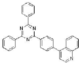
[화학식 18]
