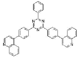
[화학식 42]
