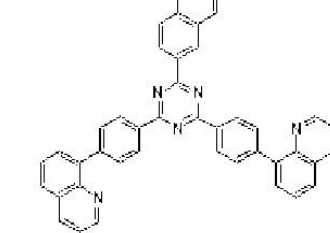
[화학식 50]
