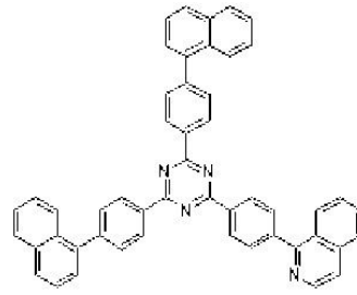
[화학식 11]
