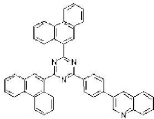
[화학식 15]
