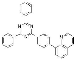
[화학식 24]
