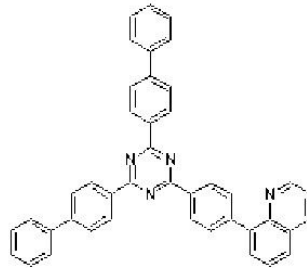
[화학식 28]
