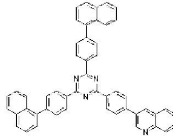
[화학식 17]
