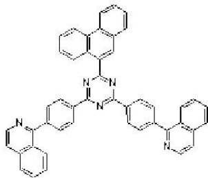
[화학식 33]
