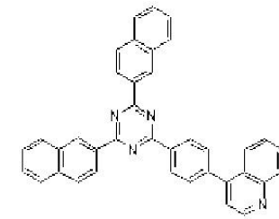
[화학식 20]
