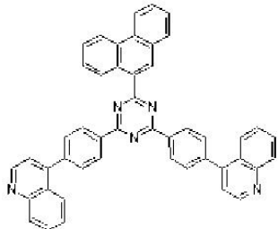
[화학식 45]
