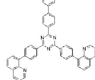
[화학식 49]
