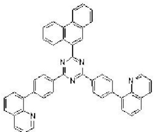
[화학식 48]
