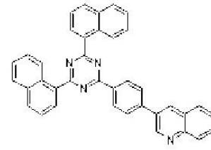
[화학식 13]
