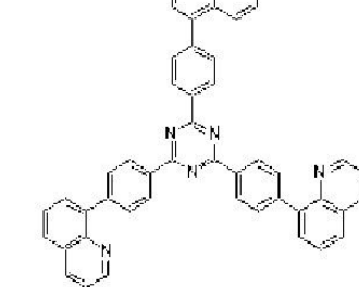
[화학식 50]
