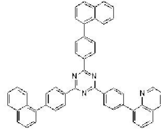
[화학식 29]
