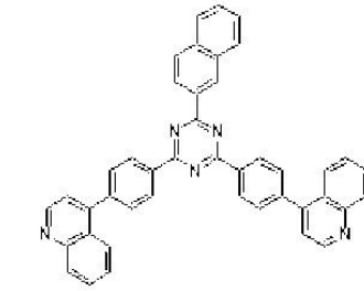
[화학식 44]
