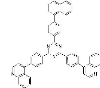
[화학식 47]
