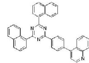
[화학식 19]
