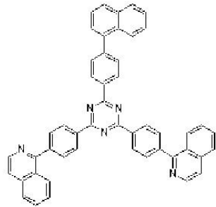
[화학식 35]
