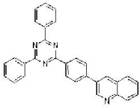
[화학식 12]
