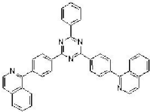
[화학식 30]
