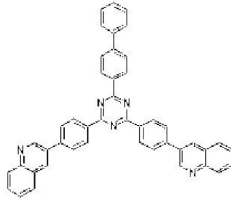
[화학식 40]
