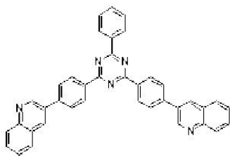
[화학식 33]
