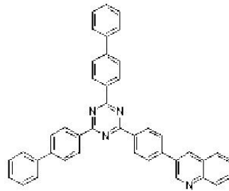
[화학식 16]
