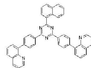
[화학식 49]
