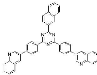
[화학식 35]
