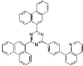
[화학식 27]
