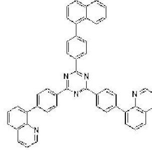
[0143] [화학식 50]
