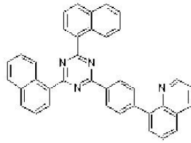
[화학식 25]
