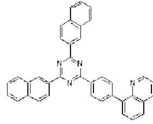
[화학식 26]
