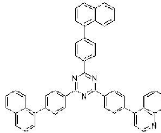
[화학식 20]
