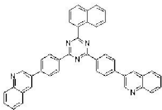
[화학식 34]
