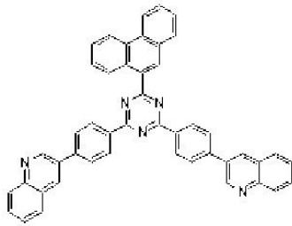
[화학식 39]
