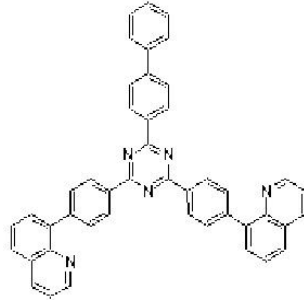
[0143] [화학식 49]
