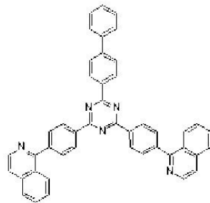
[화학식 34]
