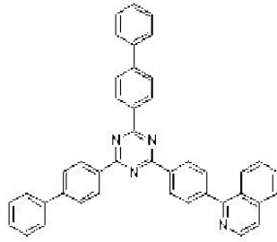
[화학식 10]
