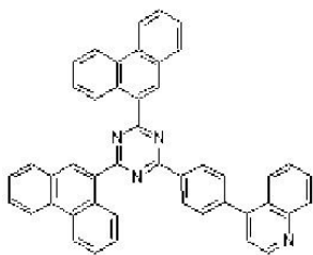
[화학식 18]
