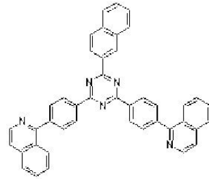
[화학식 32]
