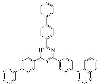
[화학식 19]
