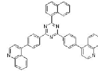
[화학식 43]
