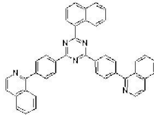
[화학식 31]
