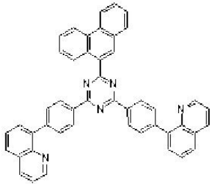
[0143] [화학식 48]
