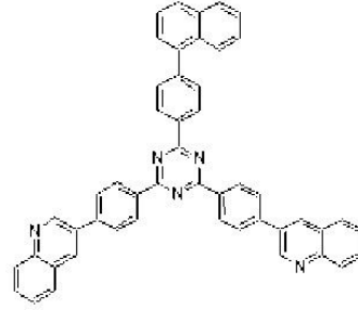
[화학식 41]
