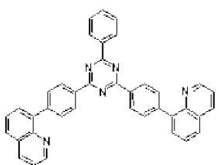
[화학식 48]
