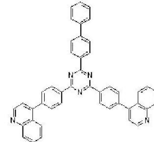
[화학식 46]
