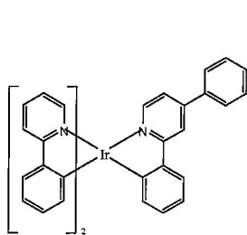
화합물 1
