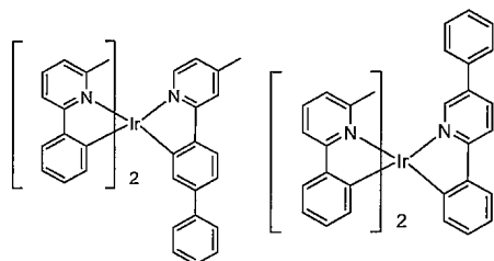
화합물 10
