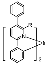
화합물 16
