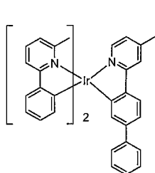
화합물 10
