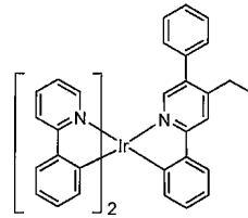
화합물 30
