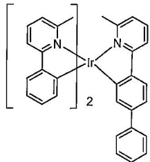
화합물 13
