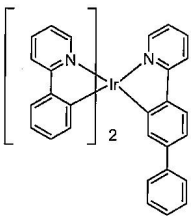
화합물 8
