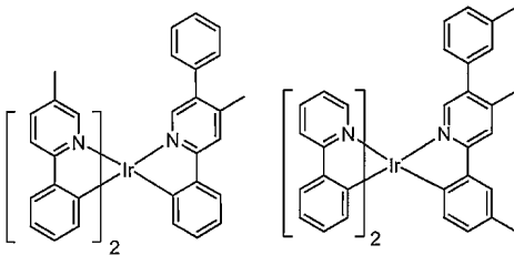
화합물 31
