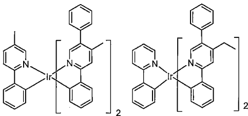
화합물 34
