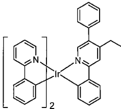
화합물 30
