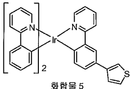
화합물 5
