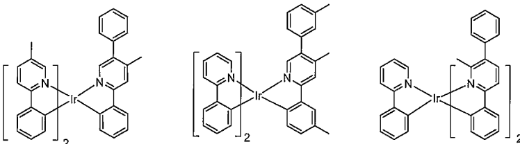
화합물 31
