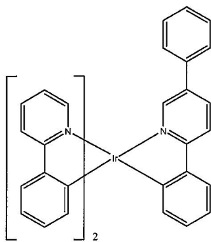
화합물 2
