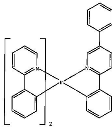
화합물 2
