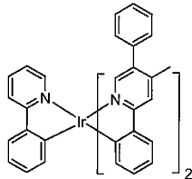
화합물 29
