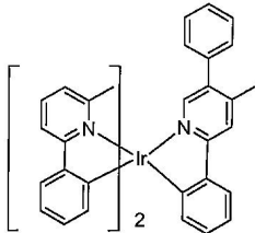
화합물 14
