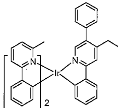
화합물 37
