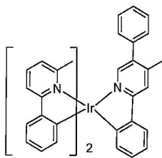
화합물 14
