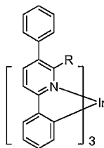
화합물 16
