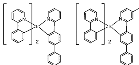
화합물 8
