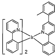
화합물 25
