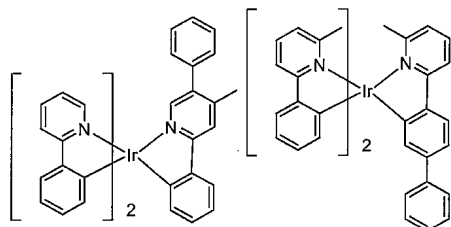
화합물 12
