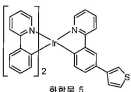
화합물 5
