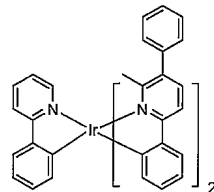
화합물 33
