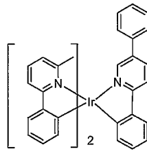
화합물 11
