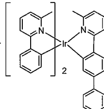
화합물 13
