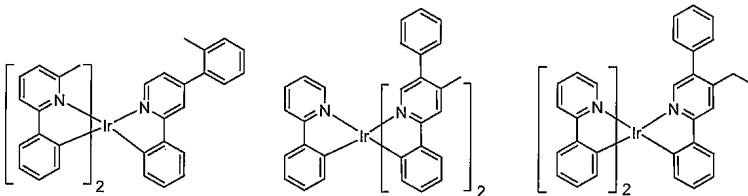
화합물 28
