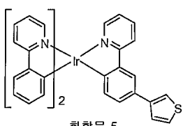
화합물 5
