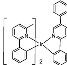
화합물 11
