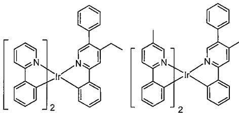
화합물 30
