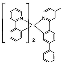
화합물 9
