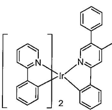
화합물 12
