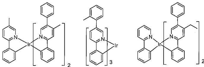
화합물 34
