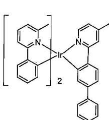
화합물 10
