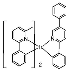
화합물 11
