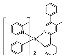
화합물 14
