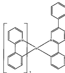
화합물 2
