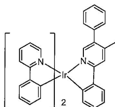
화합물 12
