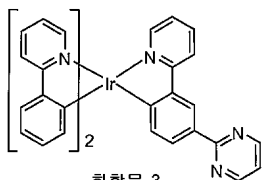
화합물 3
