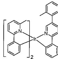
화합물 26
