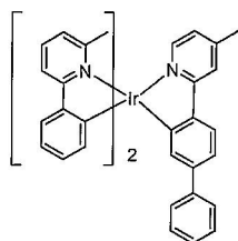
화합물 10
