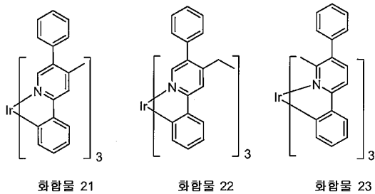
화합물 21
