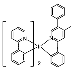
화합물 12
