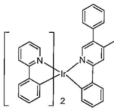
화합물 12
