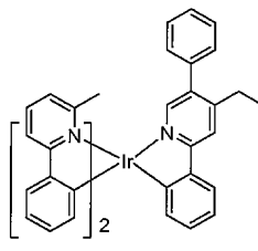
화합물 37
