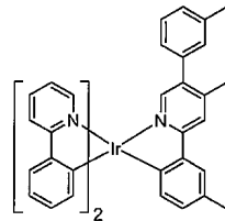
화합물 32
