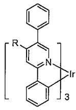
화합물 15
