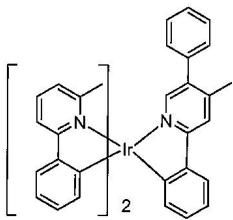
화합물 14
