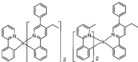
화합물 36
