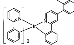
화합물 27
