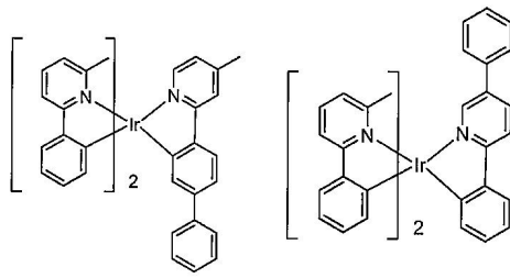
화합물 10
