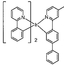
화합물 9
