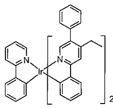
화합물 36
