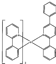
화합물 2
