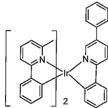
화합물 11
