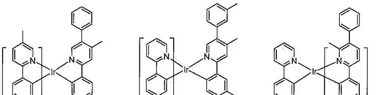
화합물 31
