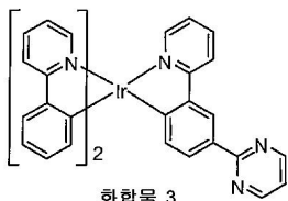
화합물 3
