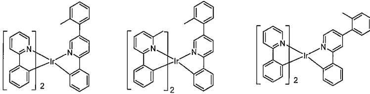
화합물 25
