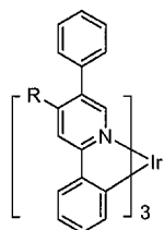
화학물 15
