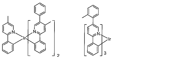
화합물 34
