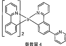
화합물 4
