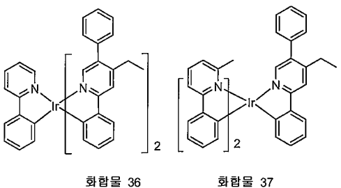
화합물 36
