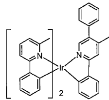
화합물 14
