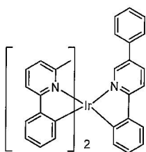
화합물 11
