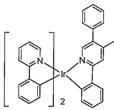
화합물 12
