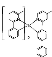
화합물 10
