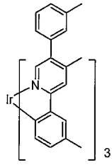
화합물 24
