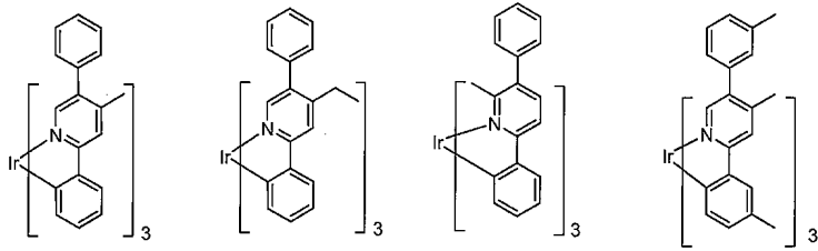
화합물 21
