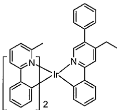
화합물 37
