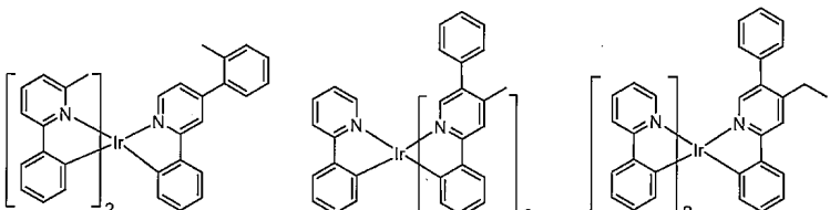
화합물 29
