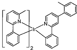
화합물 28
