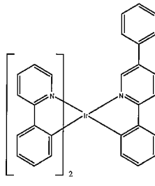
화합물 2
