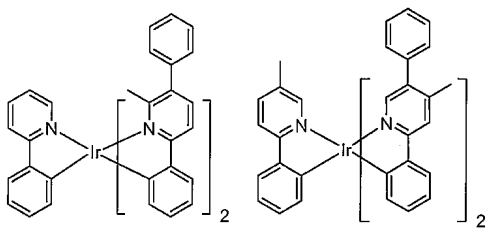
화합물 33
