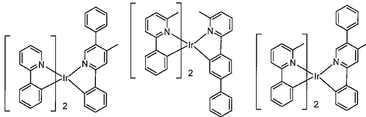
화합물 12
