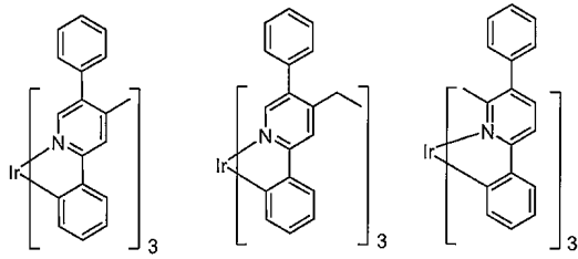
화합물 21
