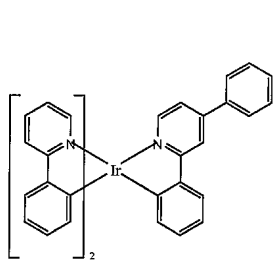
화합물 1
