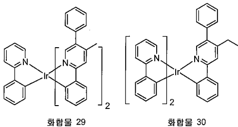
화합물 29
