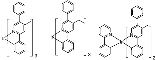
화합물 21
