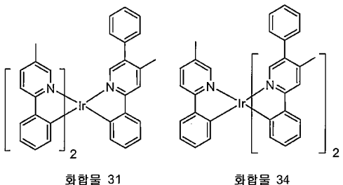
화합물 31
