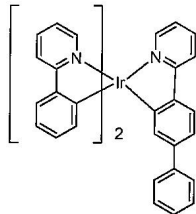
화합물 8
