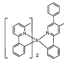
화합물 14
