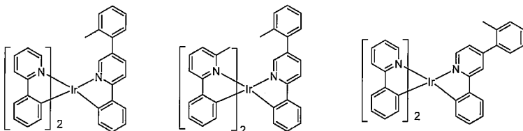
화합물 27
