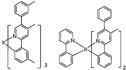
화합물 24
