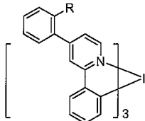
화합물 20
