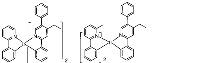
화합물 36
