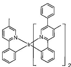
화합물 34
