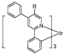
화합물 18
