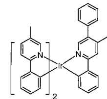
화합물 31
