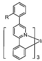
화합물 17
