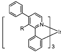
화합물 19
