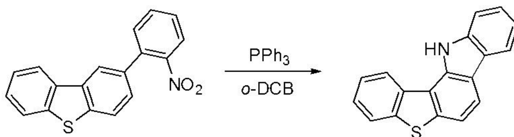
출발물질 S
