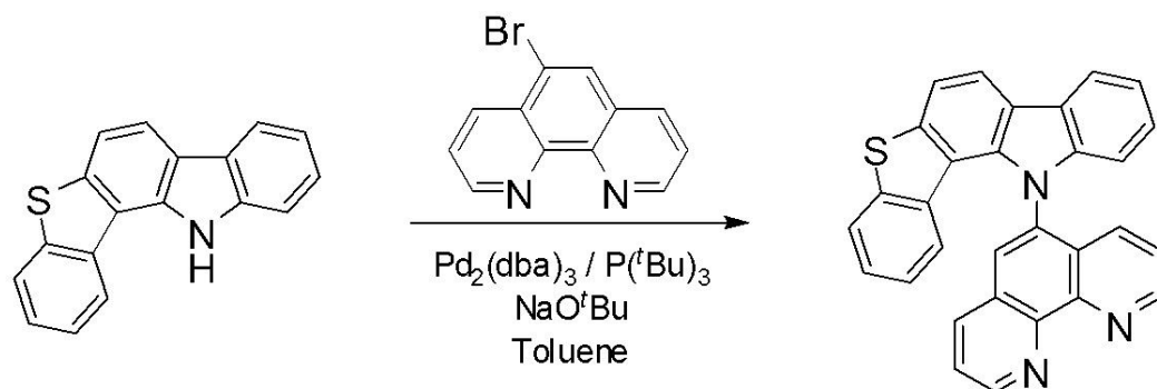
출발물질 S
