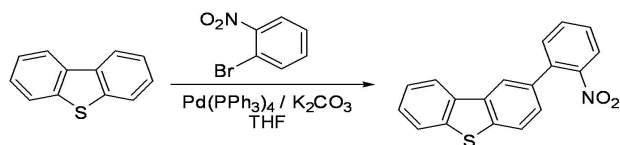
중간체 C
