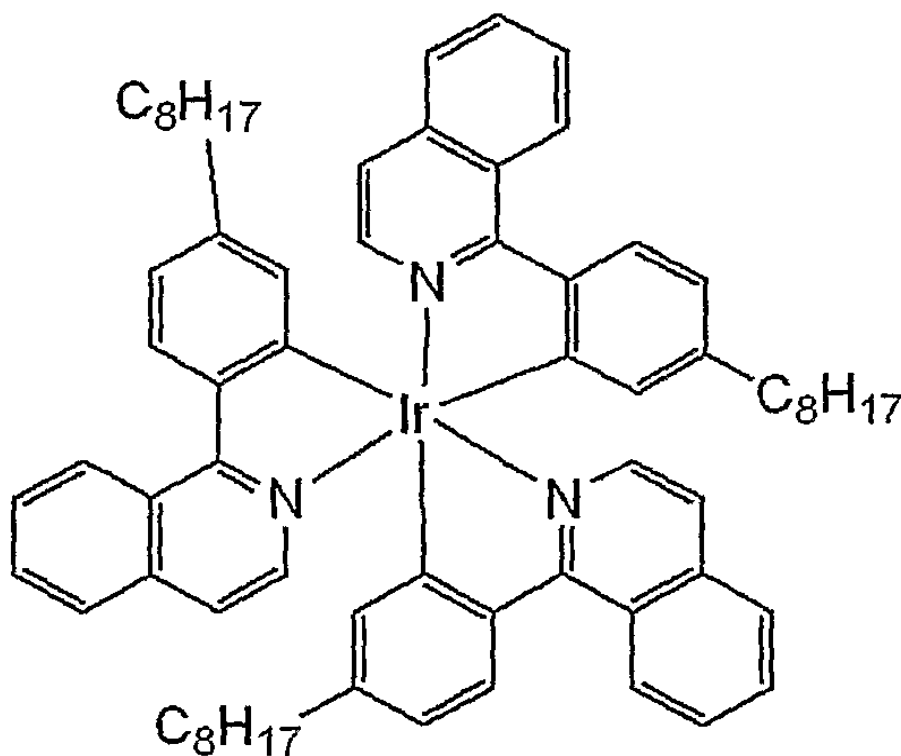
Ir(C 8 -piq) 3
