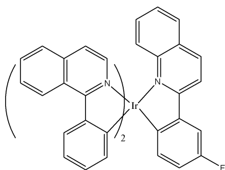
[화학식 20]
