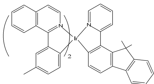
[화학식 18]
