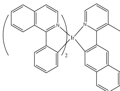
[화학식 20]
