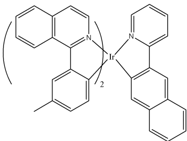
[화학식 16]
