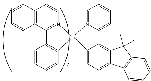
[화학식 14]
