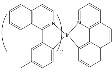
[화학식 15]
