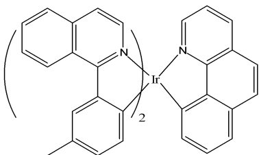
[화학식 15]
