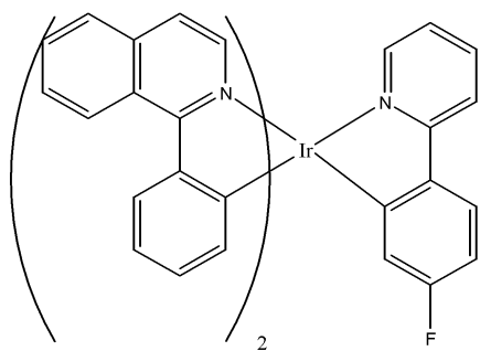
[화학식 11]
