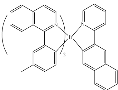
[화학식 15]
