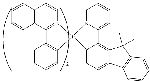
[화학식 14]
