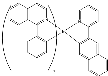
[화학식 7]
