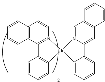
[화학식 8]
