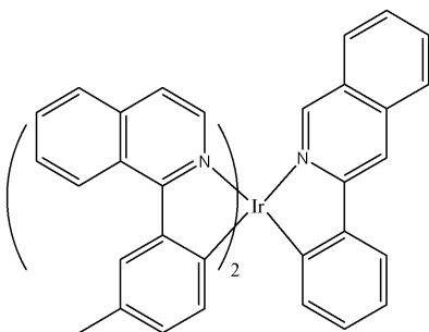
[화학식 16]
