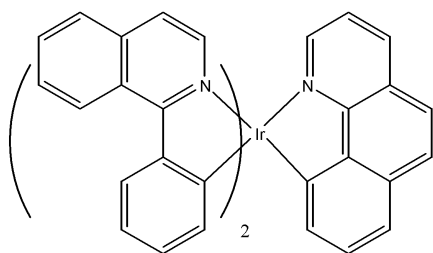
[화학식 6]
