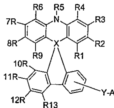
화학식 1
