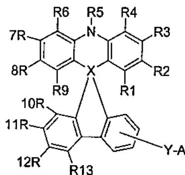
[화학식 1]
