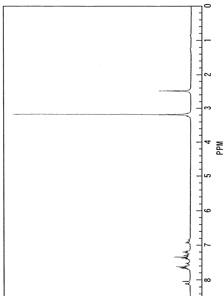
(5a)의 1 H NMR 스펙트럼
