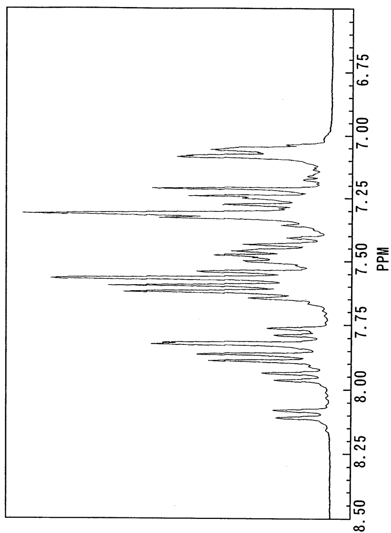
(화합물 5)의 1H NMR 스펙트럼
