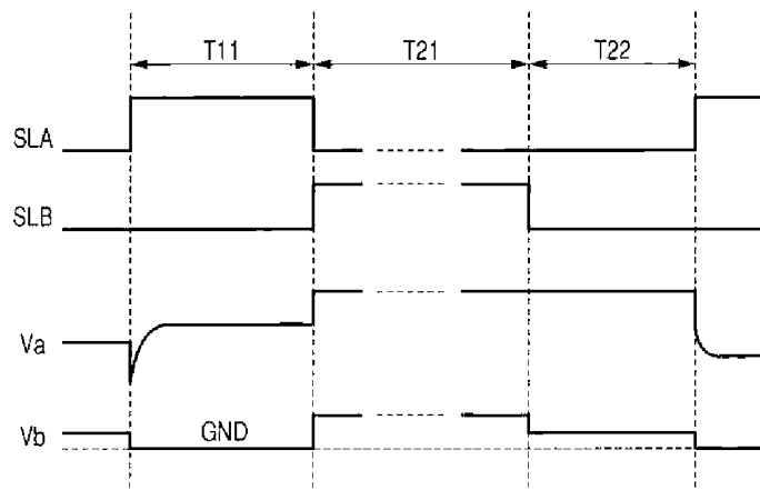
T11 ; 전류 기입 기간 T21 ; LED 구동(발광) 기간 T22 ; 흑 표시 기간
