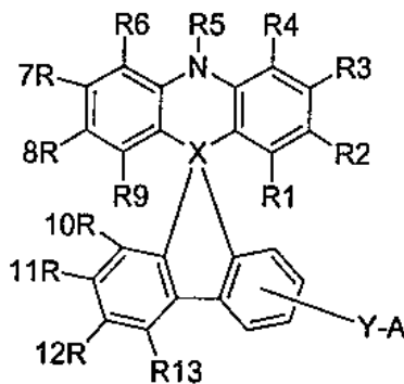
[화학식 1]
