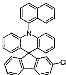
[화학식 b]
