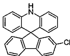
[화학식 a]
