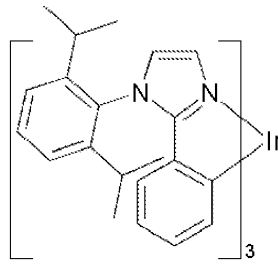
에미터 A(Emitter A)
