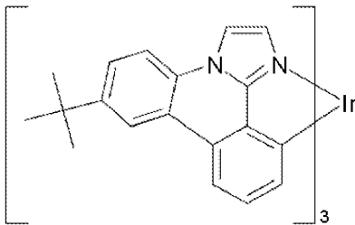
에미터 B
