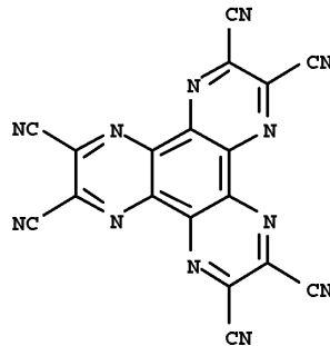
화합물 C
