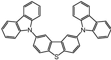
화합물 A
