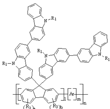
화학식 1
