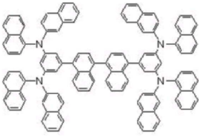
[화학식 32]
