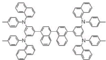
[화학식 25]
