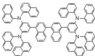
[화학식 31]
