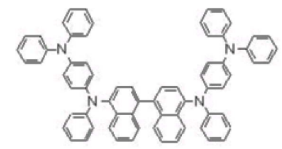
[화학식 37]
