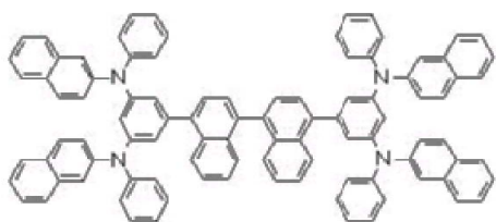
[화학식 24]
