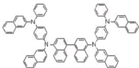
[화학식 44]
