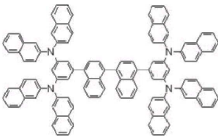
[화학식 34]
