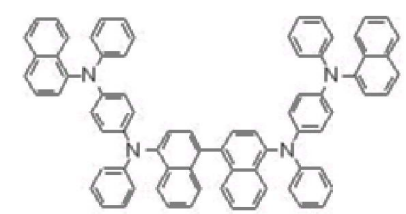
[화학식 38]
