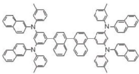
[화학식 28]
