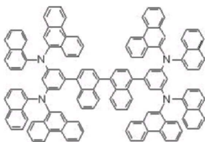
[화학식 34]
