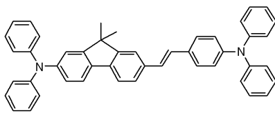
화합물 223
