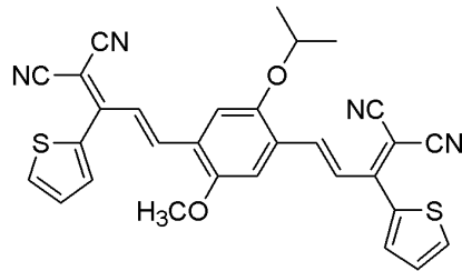
화학식 21
