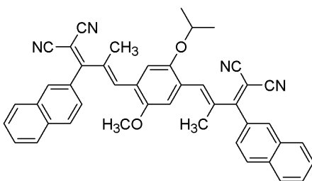
<화학식 23>
