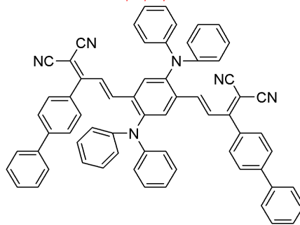
화학식 16
