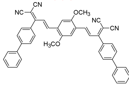
화학식 15
