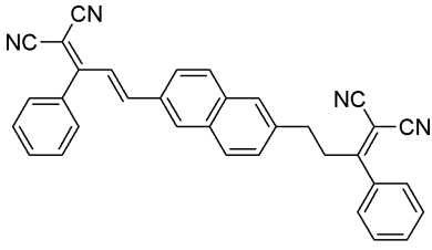
<화학식 14>
