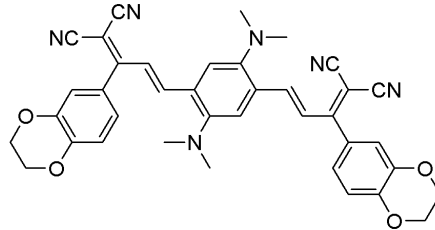
화학식 11
