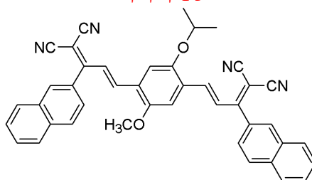
화학식 14
