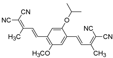
<화학식 18>
