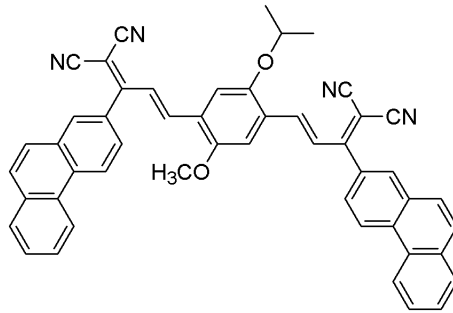
화학식 20
