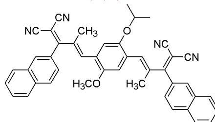
화학식 22
