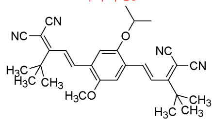
화학식 18
