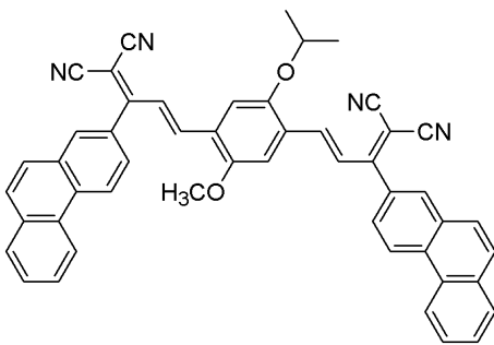
<화학식 21>
