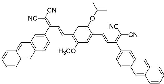
<화학식 20>
