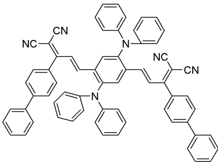
<화학식 17>
