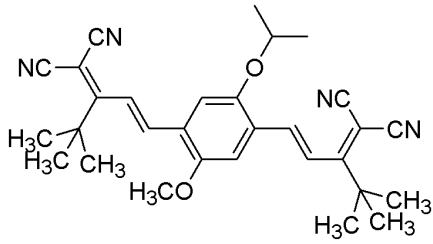
<화학식 19>
