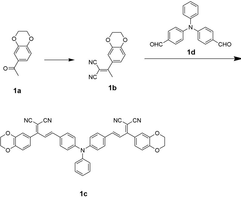
반응식 1
