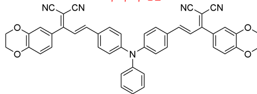
화학식 12
