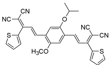
<화학식 22>
