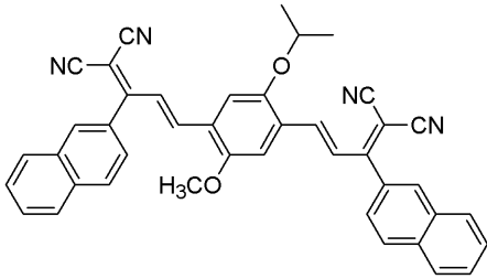
<화학식 15>
