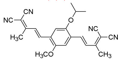
화학식 17
