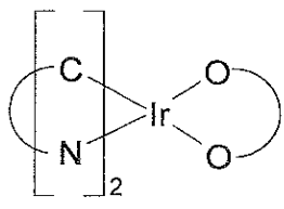
화학식 1
