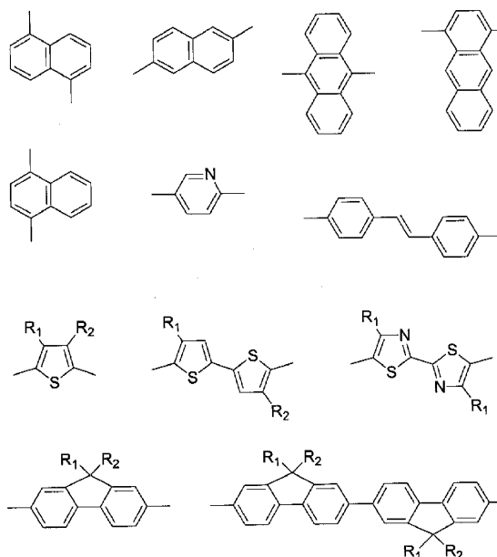
화학식 3
