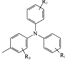
화학식 5
