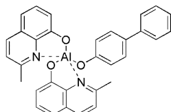
BALq
