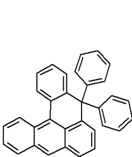
<41> <화학식 5>
