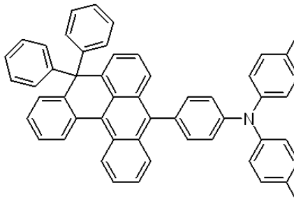
<화학식 14>
