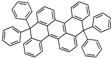
<화학식 13>
