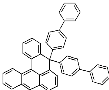
<화학식 6>
