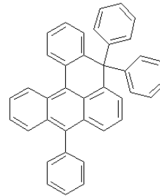
<화학식 28>
