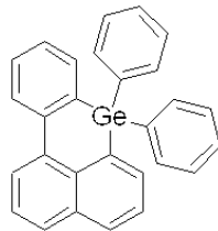
<화학식 24>
