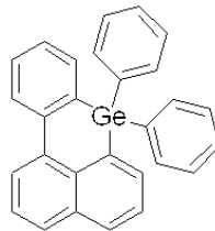
<화학식 24>
