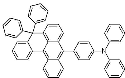
<화학식 13>
