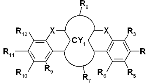
<화학식 2b>
