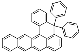
<화학식 7>
