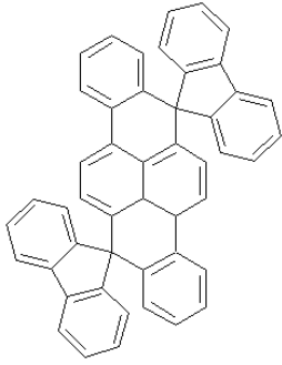
<화학식 25>
