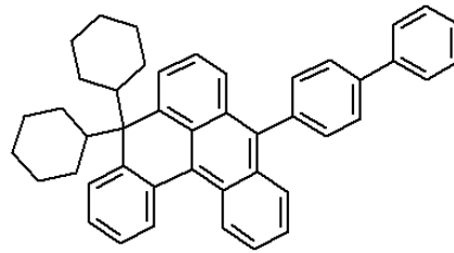
<화학식 12>
