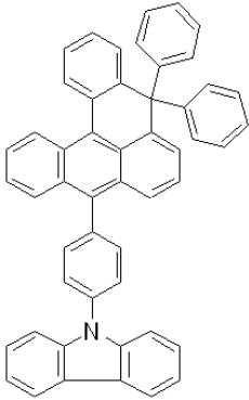
<화학식 27>
