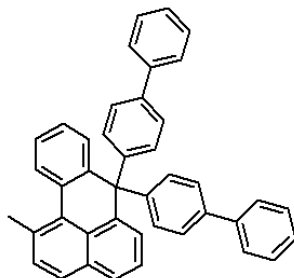
<화학식 4>
