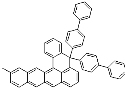
<화학식 22>
