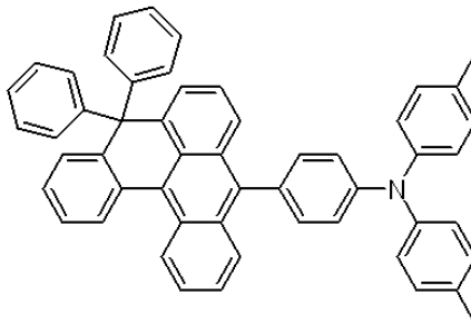
<화학식 14>
