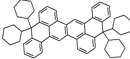
<화학식 10>
