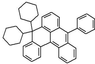
<화학식 11>
