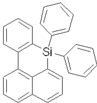
<화학식 23>
