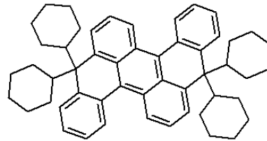
<화학식 14>
