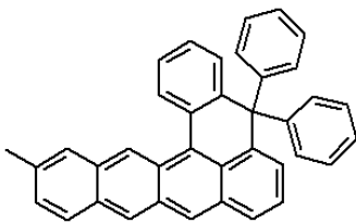
<화학식 21>
