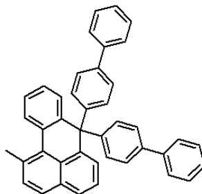
<화학식 4>
