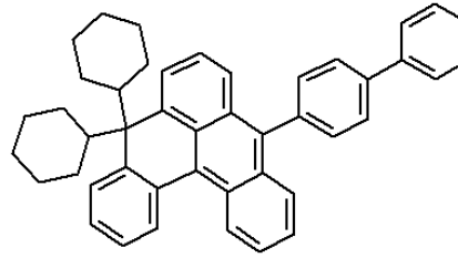
<화학식 12>
