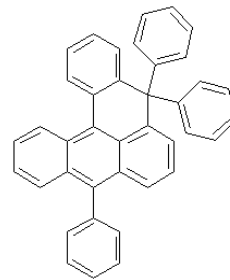
<화학식 28>
