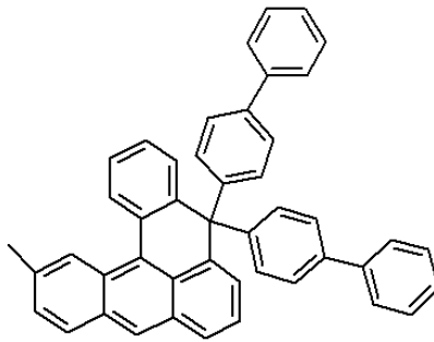
<화학식 20>
