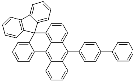
<화학식 18>
