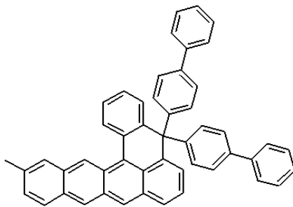
<화학식 22>
