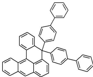
<화학식 6>
