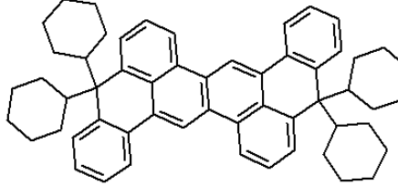
<화학식 10>
