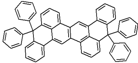
<화학식 9>
