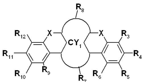
<화학식 2b>
