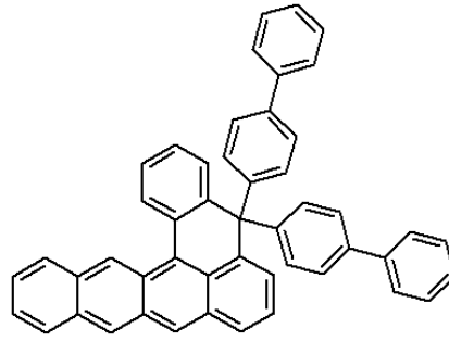
<화학식 8>
