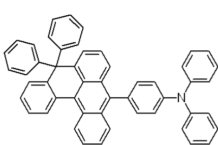
<화학식 13>
