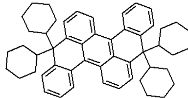
<화학식 14>
