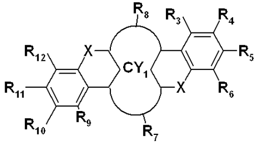
<화학식 2a>
