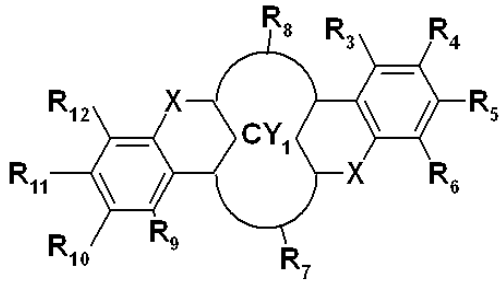
<30> <화학식 2a>
