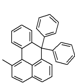
<화학식 3>
