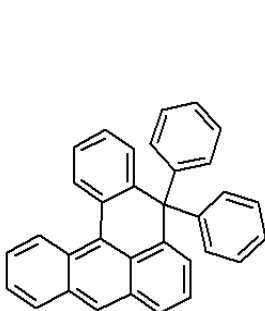
<화학식 5>
