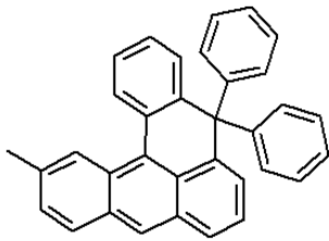
<화학식 19>
