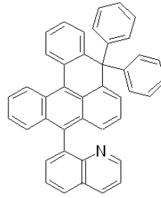
<화학식 26>
