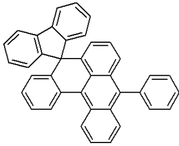
<화학식 17>
