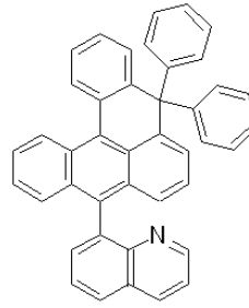
<화학식 26>
