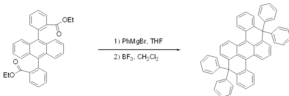
화합물 13
