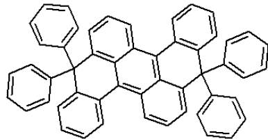
<화학식 13>
