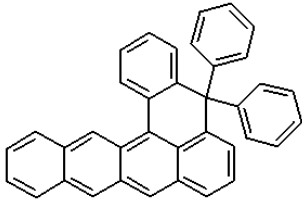
<화학식 7>
