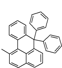
<39> <화학식 3>
