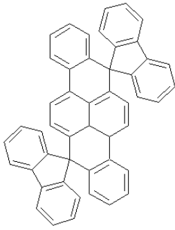
<화학식 25>
