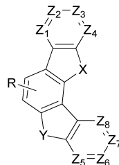
[화학식 6]
