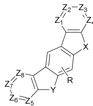
[화학식 6]
