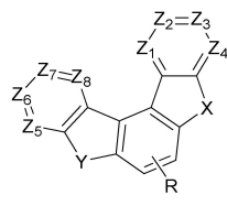
[화학식 5]
