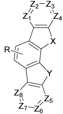
[화학식 5]
