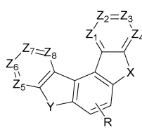
[화학식 5]
