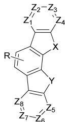
[화학식 5]
