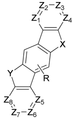
[화학식 4]
