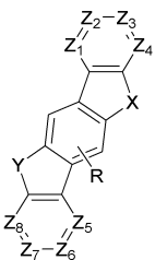
[화학식 4]
