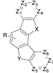
[화학식 6]
