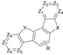
[화학식 4]
