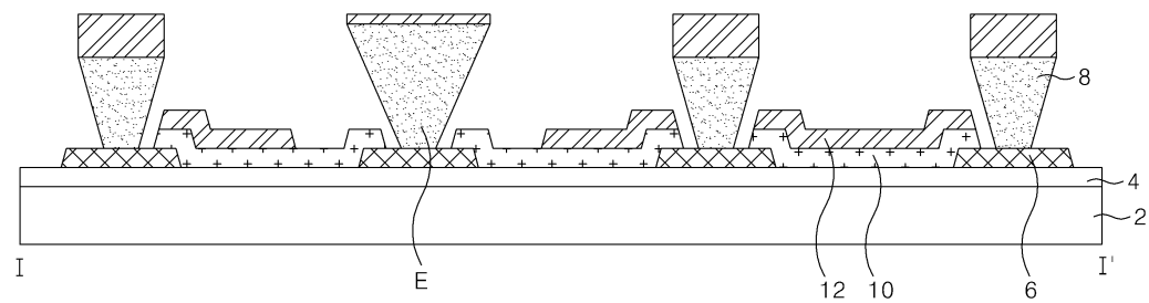
도면3b
