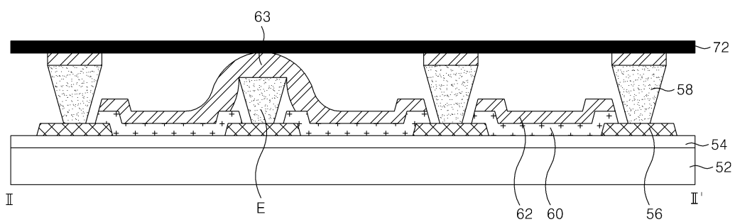
도면6
