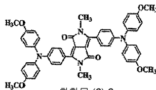
화합물 (6)-3
