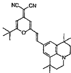
화합물 (8)-2
