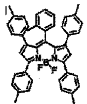
화합물 (7)-37
