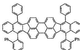
화합물 (5)-8
