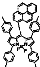
화합물 (7)-54
