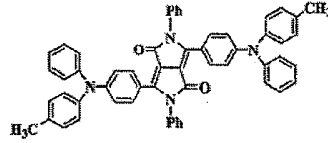
화합물 (6)-10
