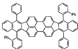
화합물 (5)-7
