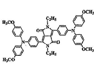
화합물 (6)-5
