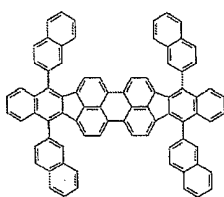
화합물 (5)-6
