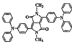
화합물 (6)-1
