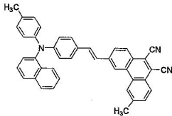
화합물 (9)-21
