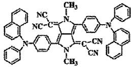
화합물 (6)-11
