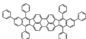
화합물 (5)-3
