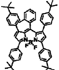
화합물 (7)-37
