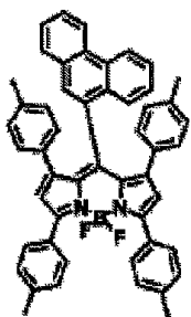
화합물 (7)-53
