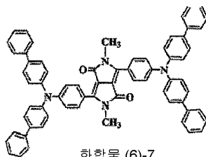
화합물 (6)-7
