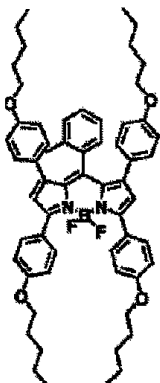
화합물 (7)-40
