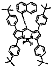
화합물 (7)-67
