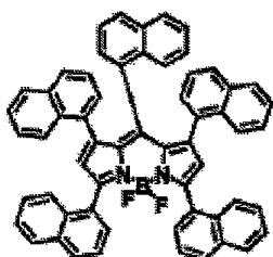
화합물 (7)-68
