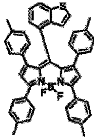
화합물 (7)-61
