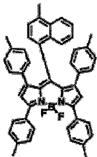
화합물 (7)-58
