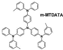
구조식 (101)
