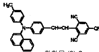
화합물 (9)-6
