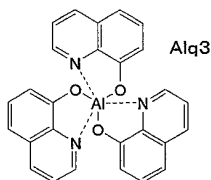
구조식 (105)
