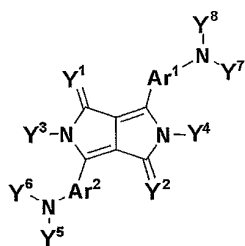
일반식 (6)
