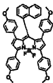
화합물 (7)-66
