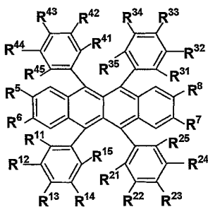
일반식 (1a)
