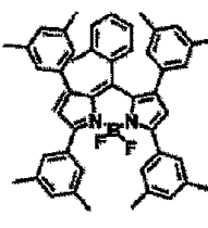
화합물 (7)-36
