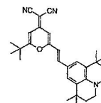
화합물 (8)-2
