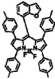
화합물 (7)-62
