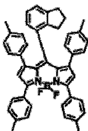
화합물 (7)-66
