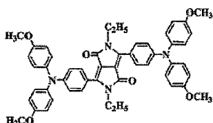
화합물 (6)-5
