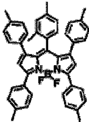
화합물 (7)-46
