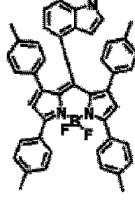
화합물 (7)-60
