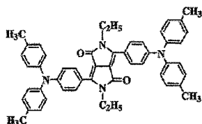
화합물 (6)-4
