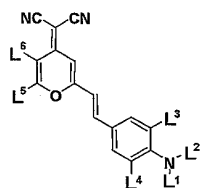
일반식 (8)
