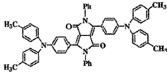
화합물 (6)-9
