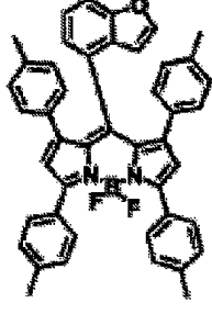
화합물 (7)-59
