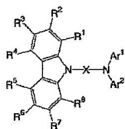
일반식 (4)
