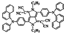
화합물 (6)-13
