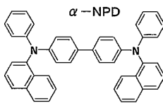
구조식 (102)
