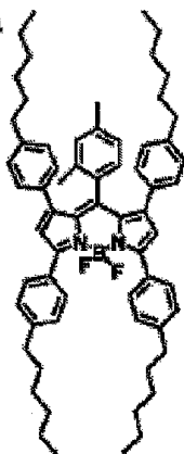
화합물 (7)-51
