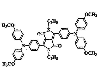
화합물 (6)-5
