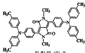
화합물 (6)-2
