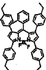
화합물 (7)-39
