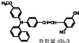
화합물 (9)-3
