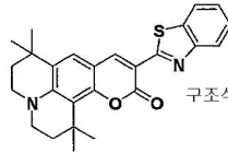
구조식 (103) ADN
