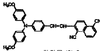
화합물 (9)-8
