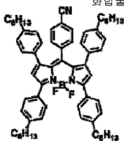
화합물 (7)-27
