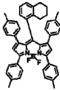
화합물 (7)-63
