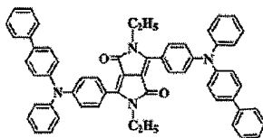
화합물 (6)-6
