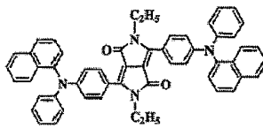
화합물 (6)-8
