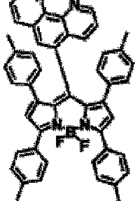
화합물 (7)-58
