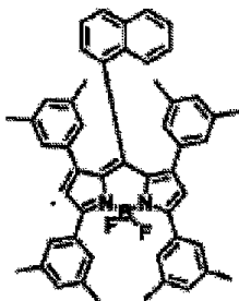
화합물 (7)-67
