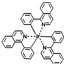
(화합물 44)
