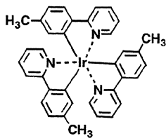
(화합물 42)
