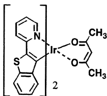
(화합물 45)
