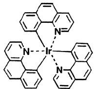
(화합물 43)
