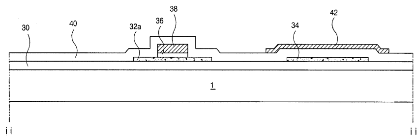
도면4d
