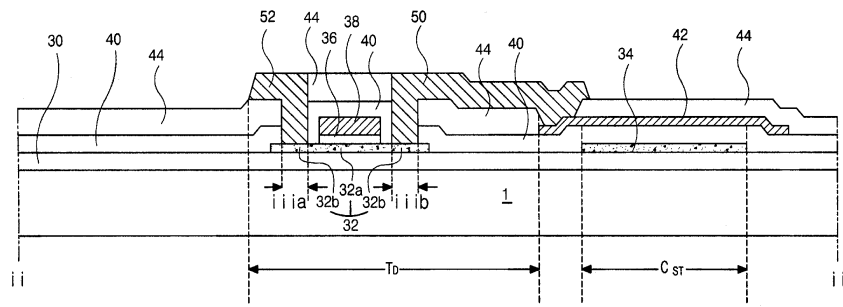
도면4f
