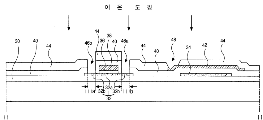
도면4d
