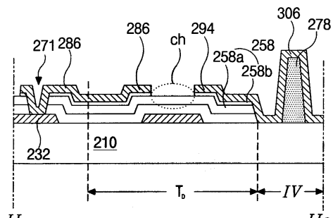
도면8d
