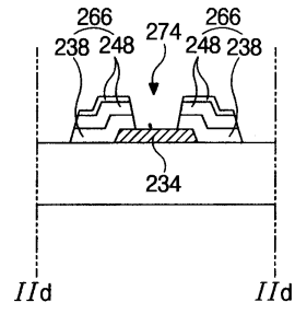
도면11c
