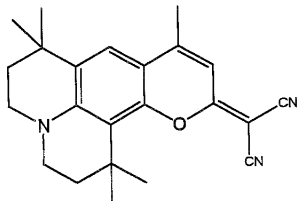
구조식 4
