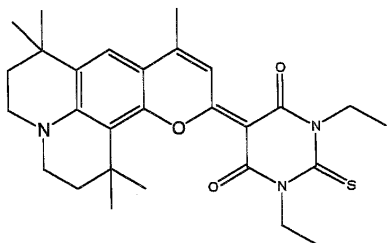
구조식 5
