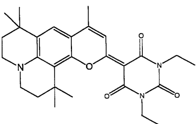
구조식 5
