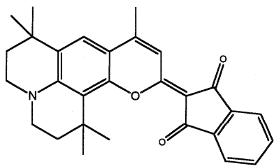
구조식 3
