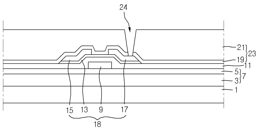
도면2c
