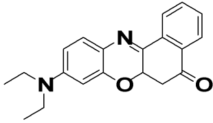
화학식 4
