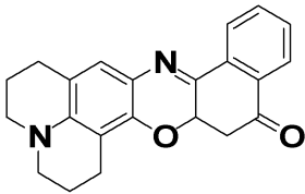
화학식 6
