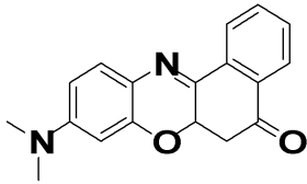
화학식 5
