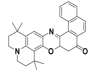
화학식 8
