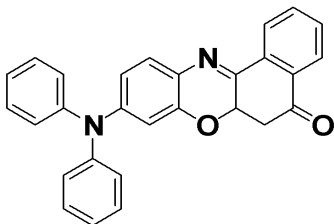
화학식 9
