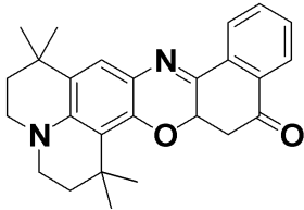
화학식 7
