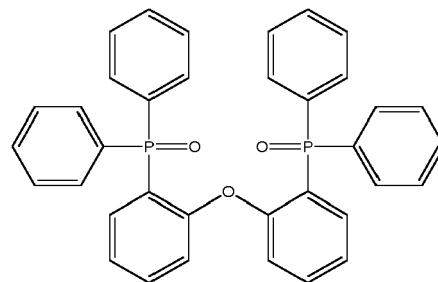
BH(DPEPO)
