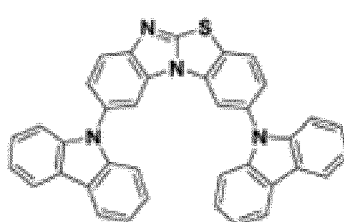
29Cz-BID-BT
