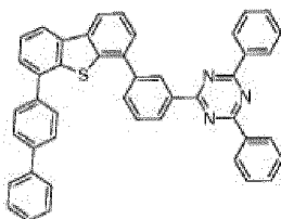
Composé C74) ;
