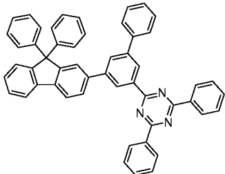
Verbindung B4
