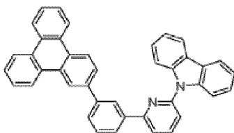
(Composé E30,
