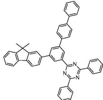
Verbindung B3
