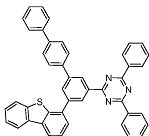
Compound A5
