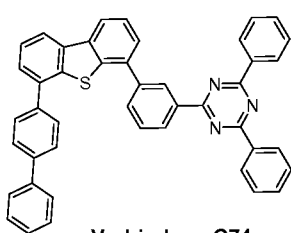
Verbindung C74
