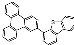
Verbindung E2
