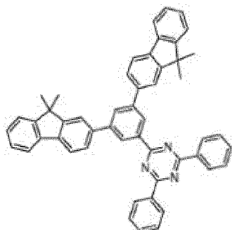
Composé B7,
