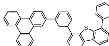
Verbindung E8
