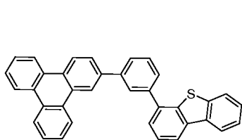
Verbindung E5
