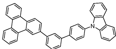
Verbindung E29
