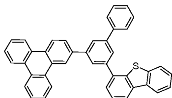
Compound E11
