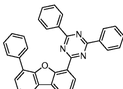
Verbindung C1
