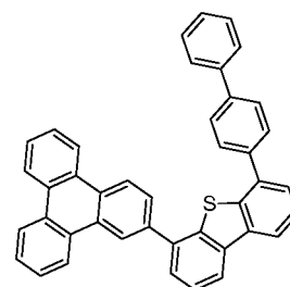
Compound E17
