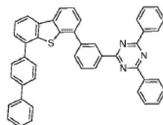
Composé C74) ;
