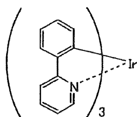
Ir(ppy) 3
