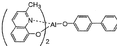
Balq
