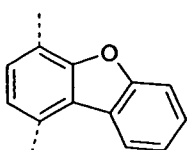
Ar S -11
