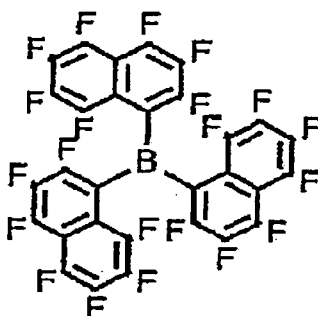
PNB
