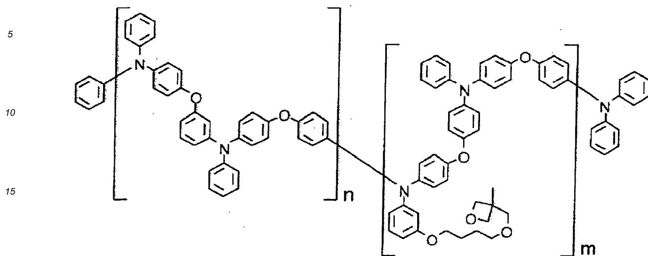
[Formula 36]
