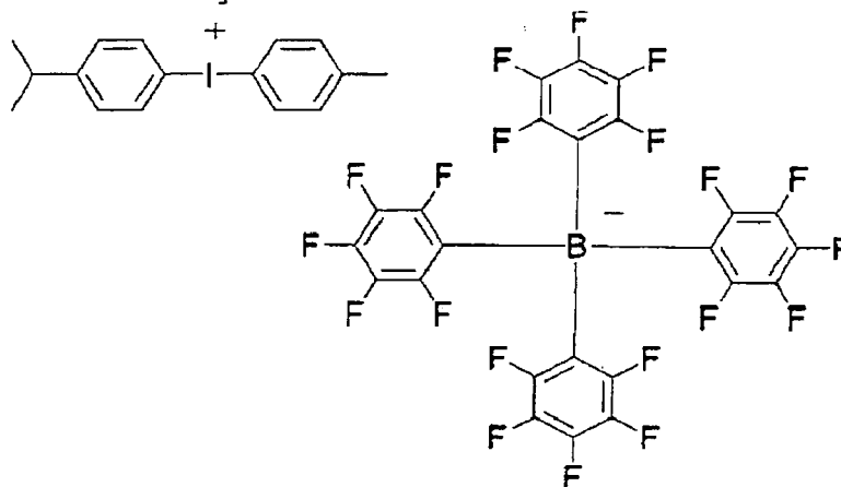
[Formula 54]
