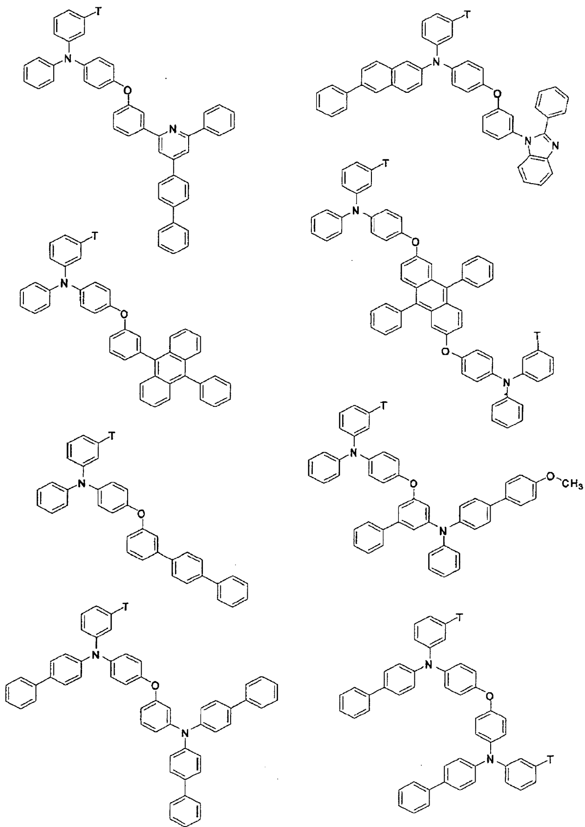
[Formula 18]
