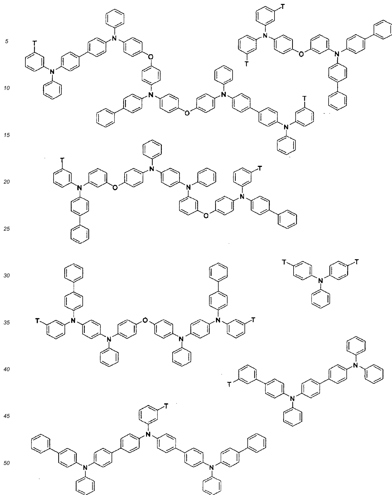
[Formula 23]
