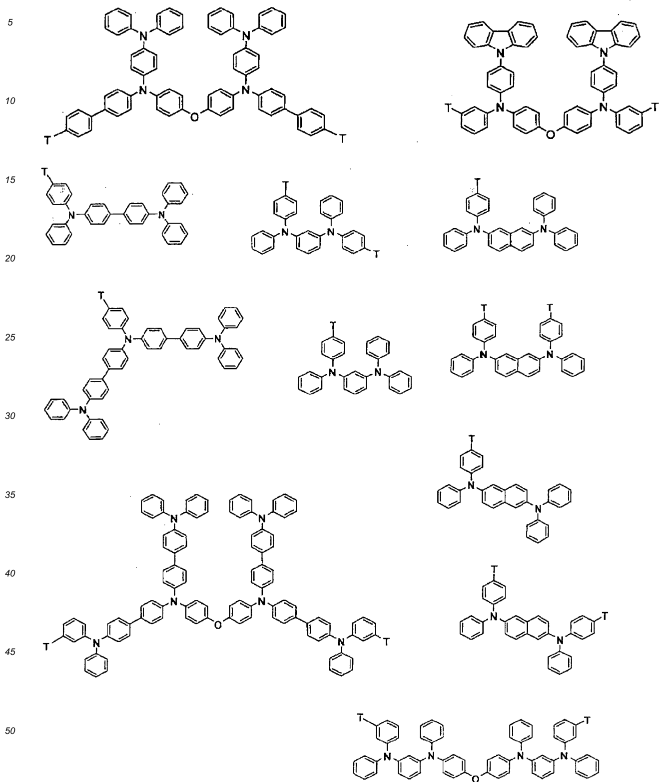
[Formula 26]
