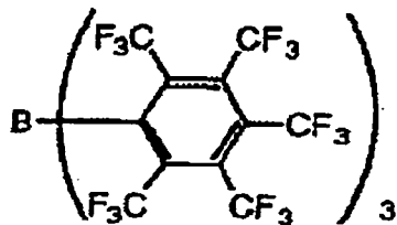
6-4
