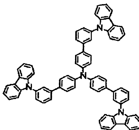
(C2)
