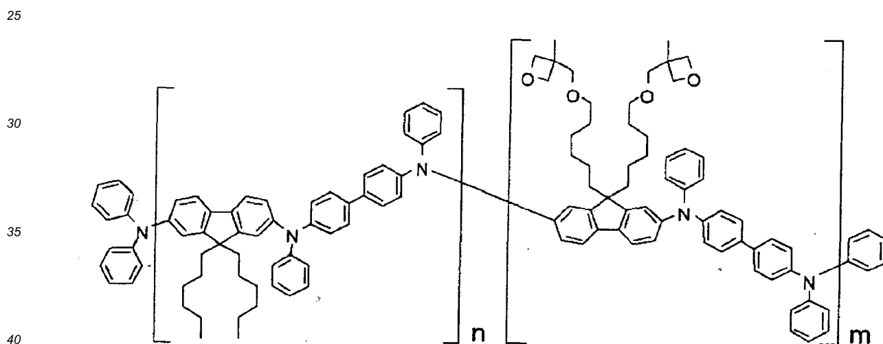
[Formula 37]
