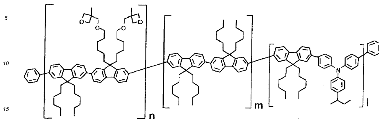
[Formula 38]
