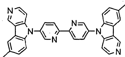
[Chem. 220]
