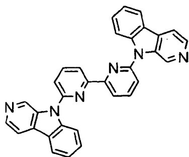
[Chem. 3]
