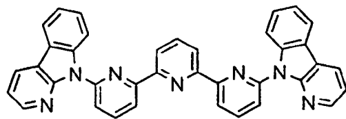
[Chem. 6]
