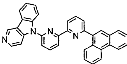
[Chem. 55]
