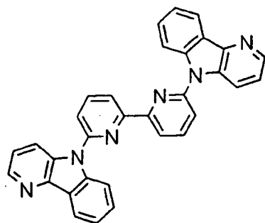
[Chem. 6]
