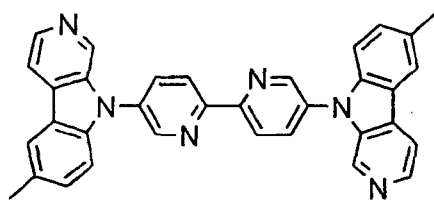
[Chem. 220]
