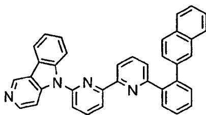
[Chem. 25]
