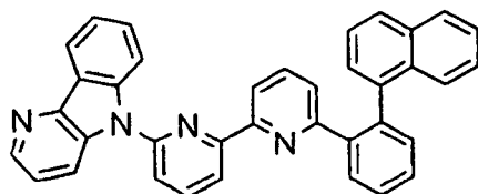
[Chem. 23]
