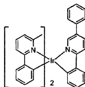
Verbindung 11
