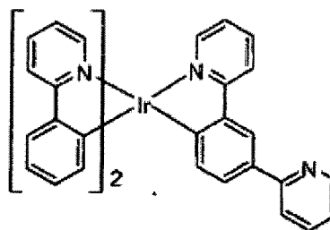
Composé 4
