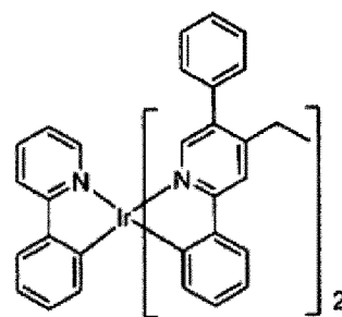
Composé 36
