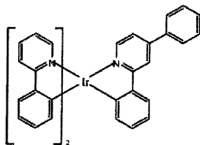
Composé 1
