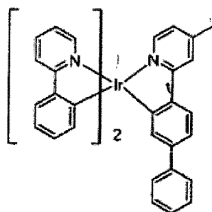
Verbindung 9
