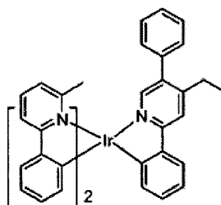
Verbindung 37
