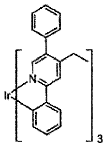
Composé 22
