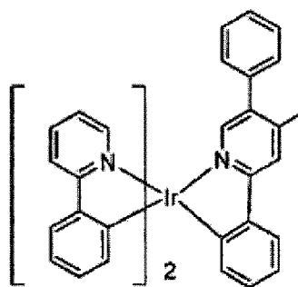
Composé 12
