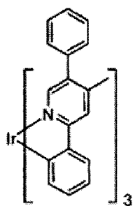
Composé 21
