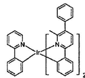
Composé 33
