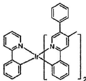
Verbindung 29
