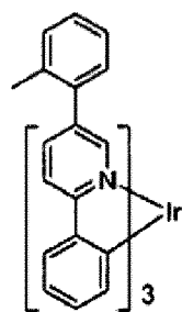
Composé 35
