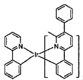
Verbindung 33
