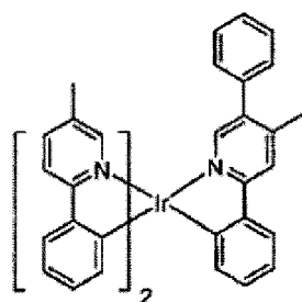
Verbindung 31
