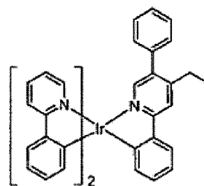
Composé 30
