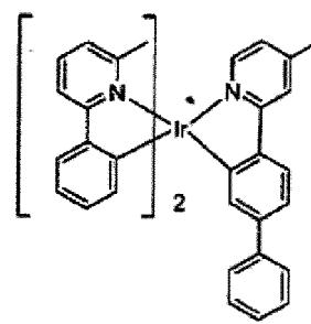
Verbindung 10
