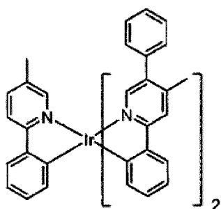
Verbindung 34
