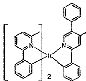
Composé 14
