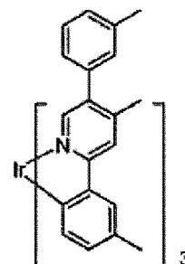
Verbindung 24
