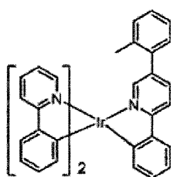
Composé 25
