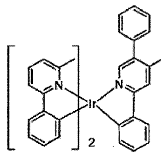
Verbindung 14
