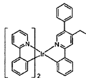
Composé 30
