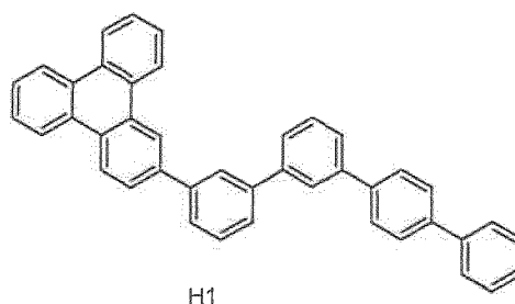
H1
