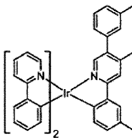
Verbindung 32
