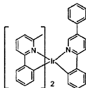
Verbindung 11
