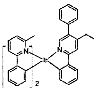
Composé 37
