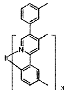
Verbindung 24
