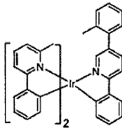
Composé 26
