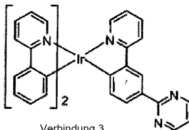
Verbindung 3
