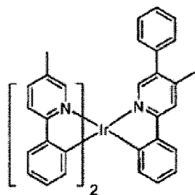
Composé 31
